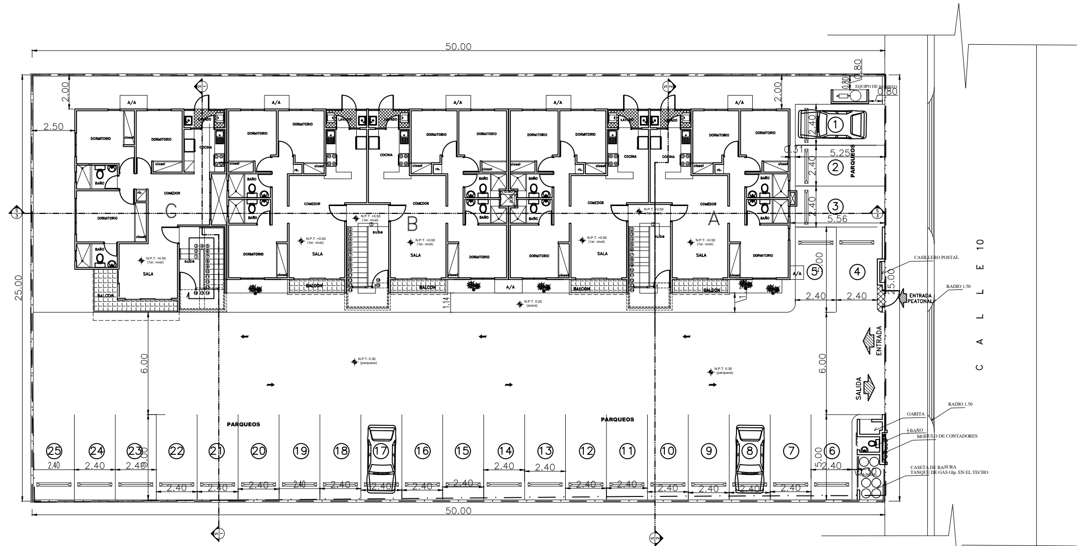
PLANTA PRIMER NIVEL- UBICACION EN EL SOLAR esc. 1:100
